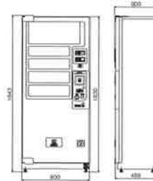
外形寸法図 (単位: mm)
